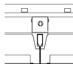
PS-2 axé sur la lumière du porteur. Raidisseur VAK 60.
