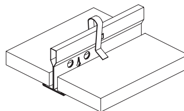
Cavalier anti-soulèvement V16K traité pour milieu humide, pour panneaux de 6 à 16 mm.
