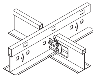
Epaulement de l'entretoise sur le porteur.
